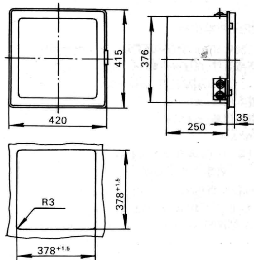
开孔尺寸
